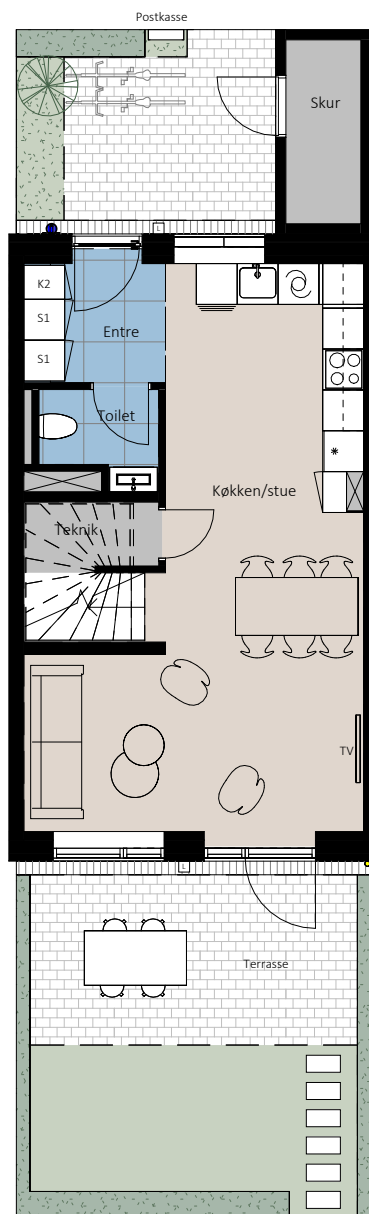
Stueplan
