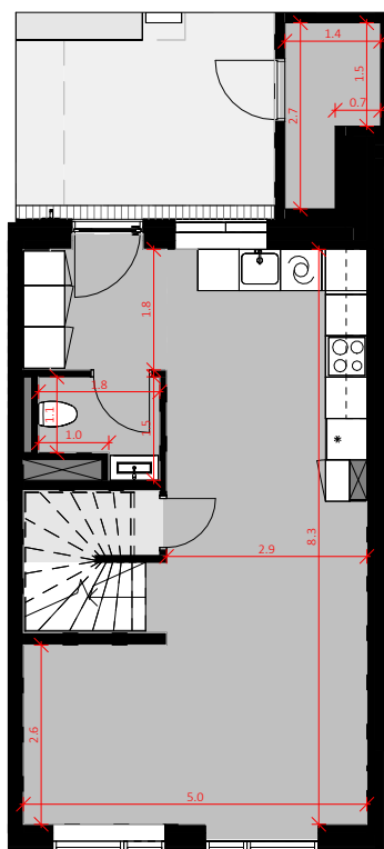
Stueplan
