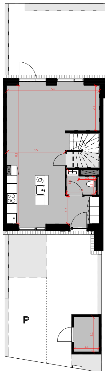
Stueplan
