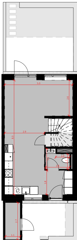
Stueplan
