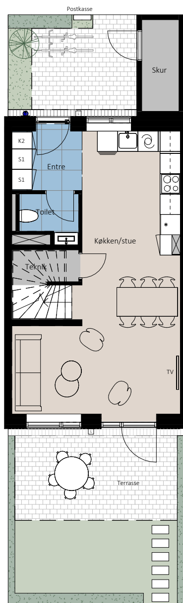
Stueplan
