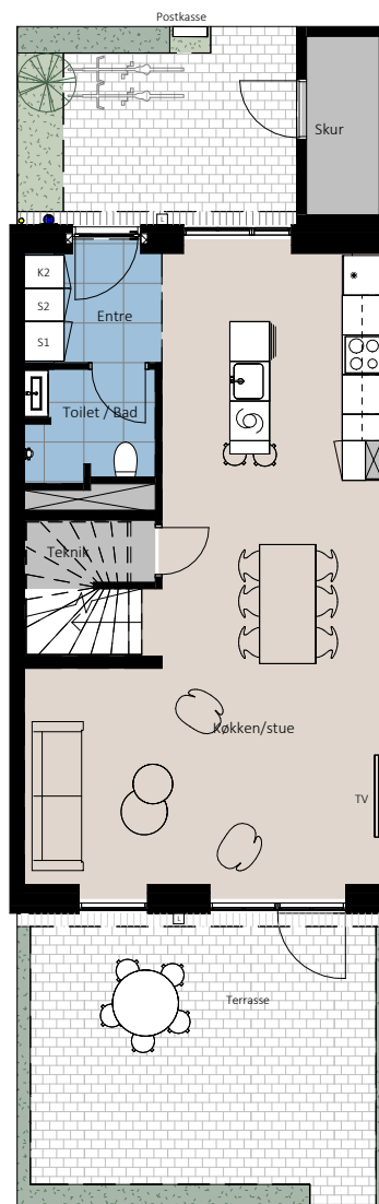
Stueplan
