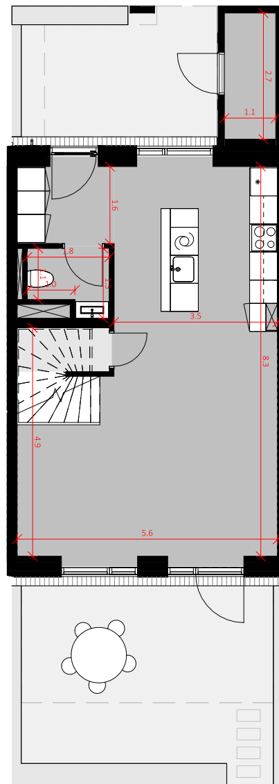
Stueplan
