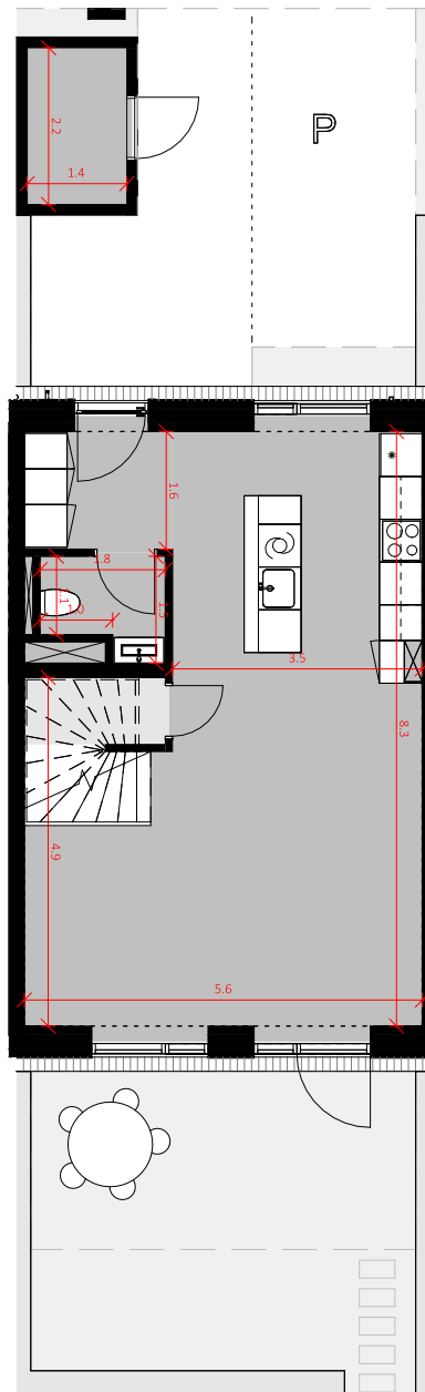
Stueplan
