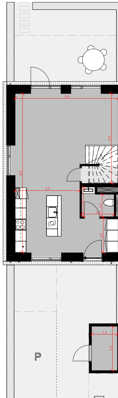
Stueplan
