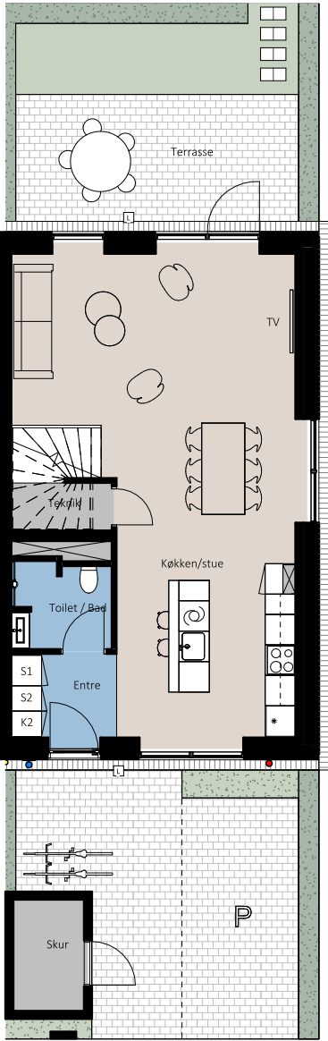
Nord Stueplan
